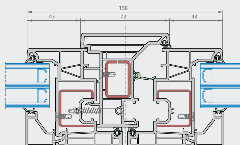
Secțiune orizontală
