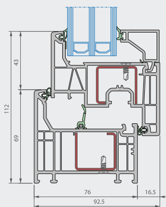
Secțiune verticală
